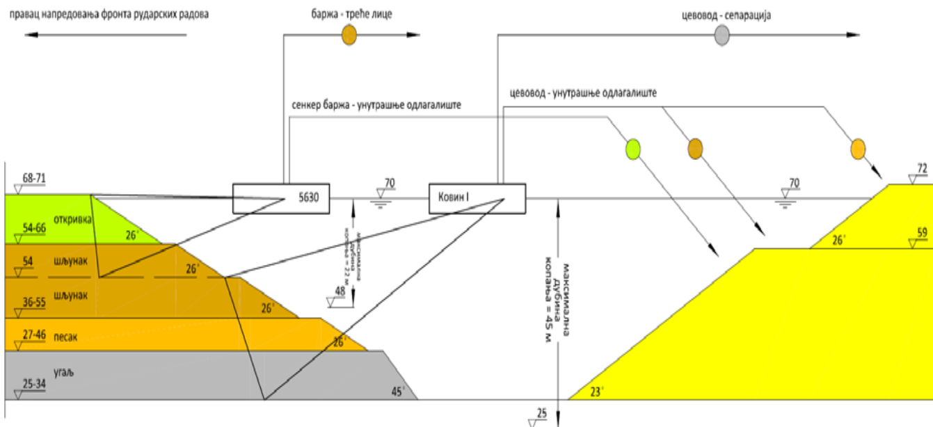
Slika 1. Принципијелна шема система експлоатације угља и шљунка на подводном копу Ковин
